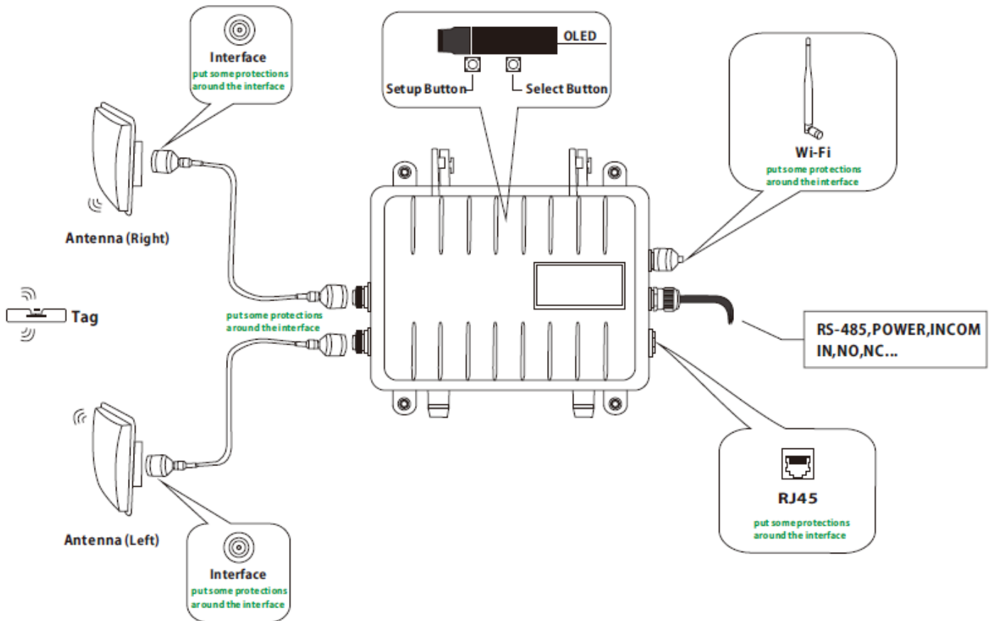
WSUHFRFIDIP6 Wiring_Diagram
