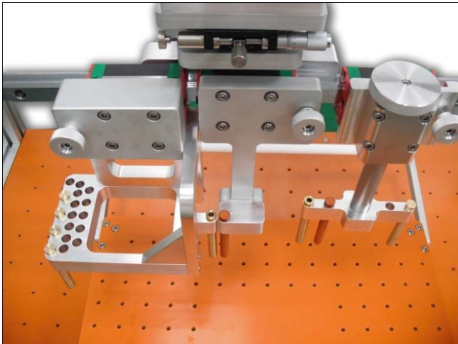
雙指劃線治具:
