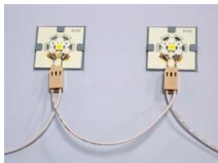
模組化燈蕊: 僅需更換單一故障晶片
