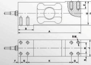
主要外形尺寸 Main Dimensions and Accessories
