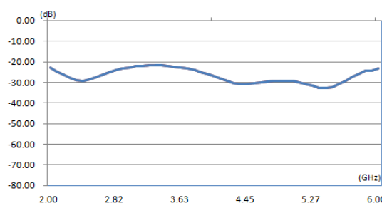
RF1 & RF2 Isolation
