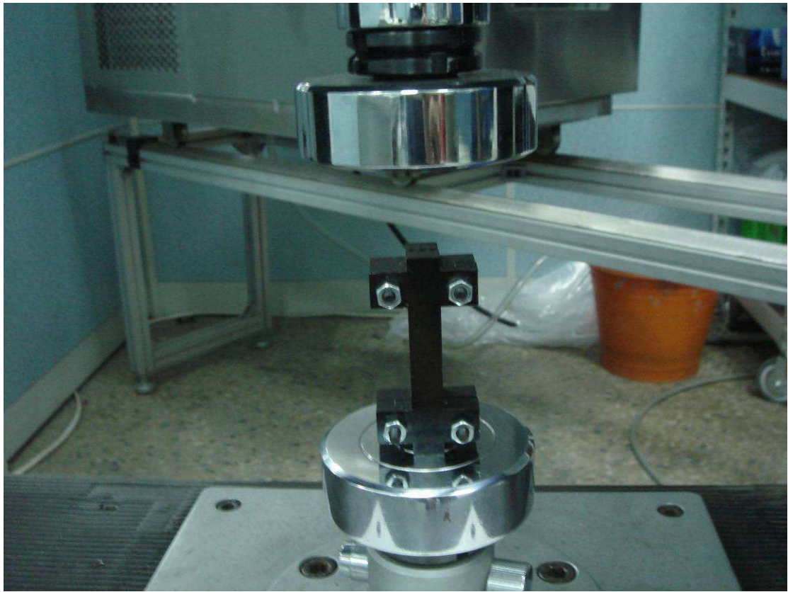
壓縮強度試驗機及治具
