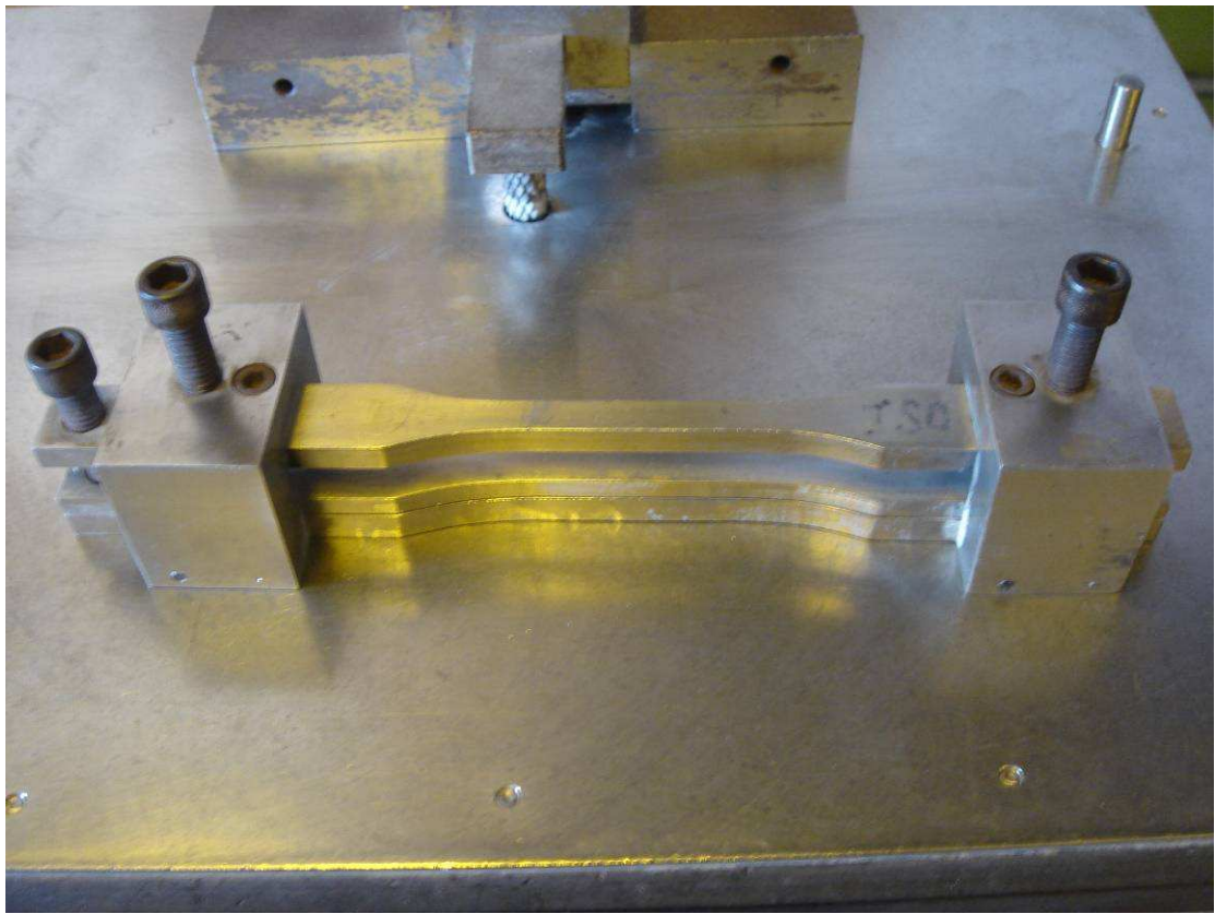
試片削成機及拉伸試片模具
