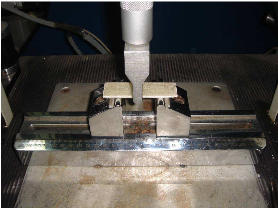
抗曲強度試驗機及治具
