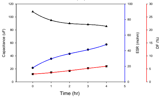
120 μF 50V 10x12mm 185°C 超高溫測試
