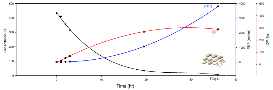
470 μF 25V 8x12mm 185°C 超高溫 40 小時破壞性測試
