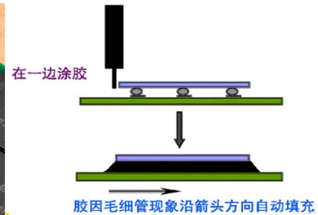
元件底部填充
