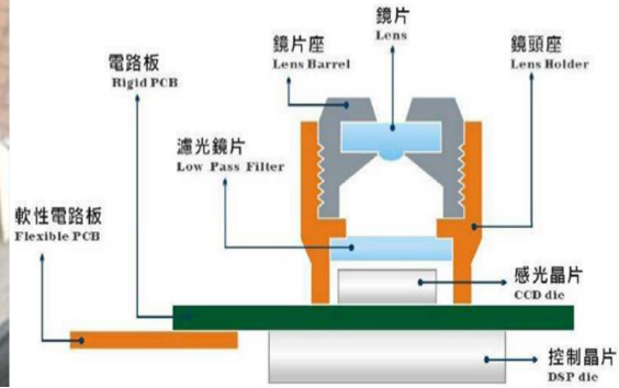
攝像頭模組封膠
