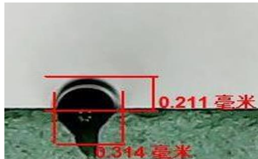
窄邊框，高寬比達到60%以上 (膠寬0.314，膠高0.211mm)
