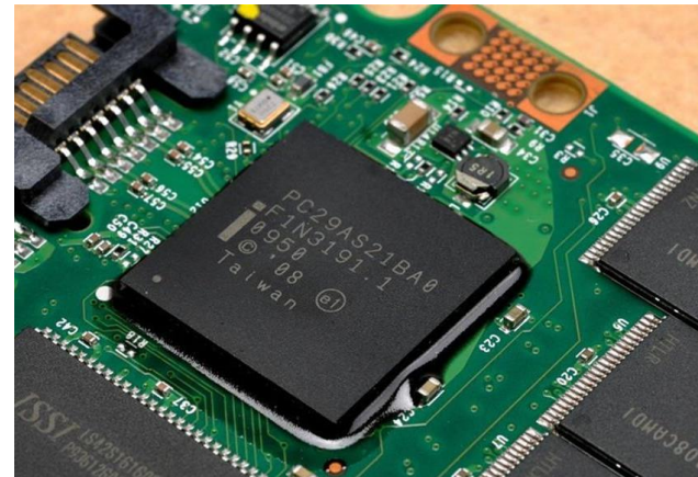
元件底部填充
