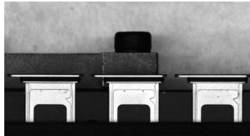
卡托防水Primer膠
