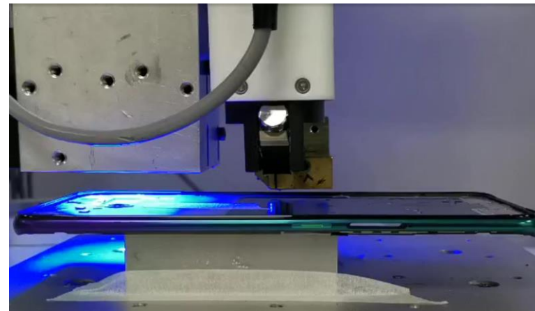
手機中框點膠
