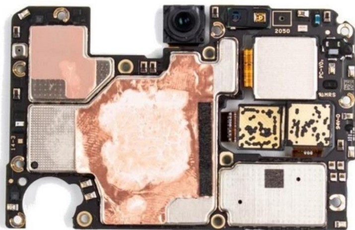
扇熱銅片點膠固定
