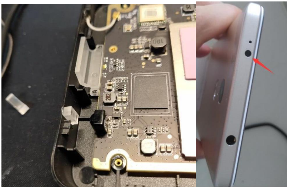
手機紅外頭點膠粘接
