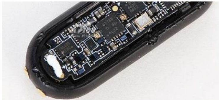
手環點熱熔膠
