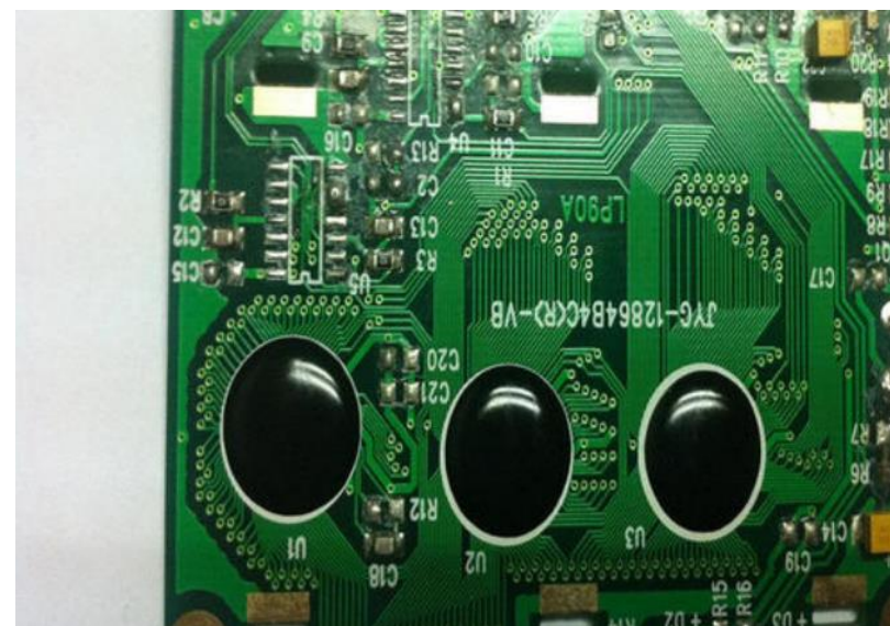
電路綁定點環氧樹脂
