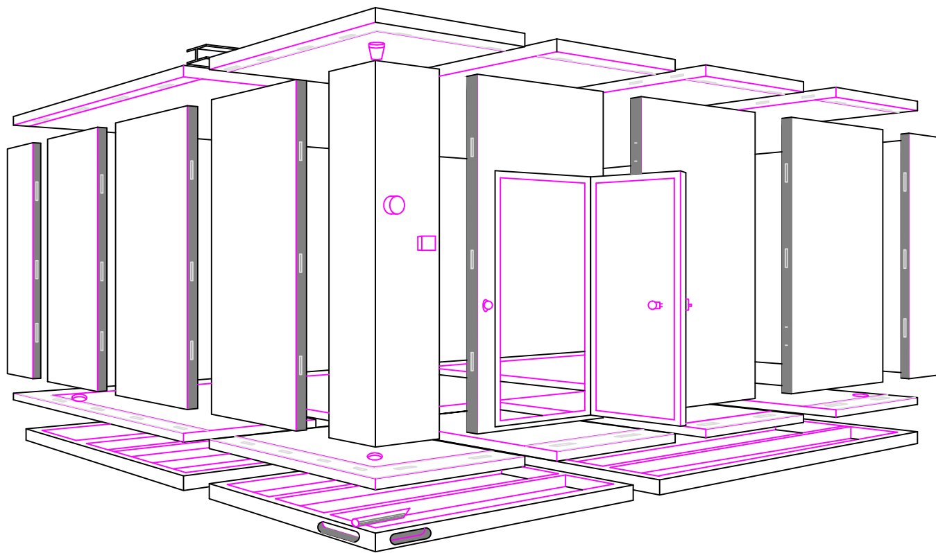
拼裝組合庫工程
