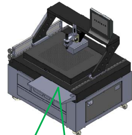
探針顯微鏡
